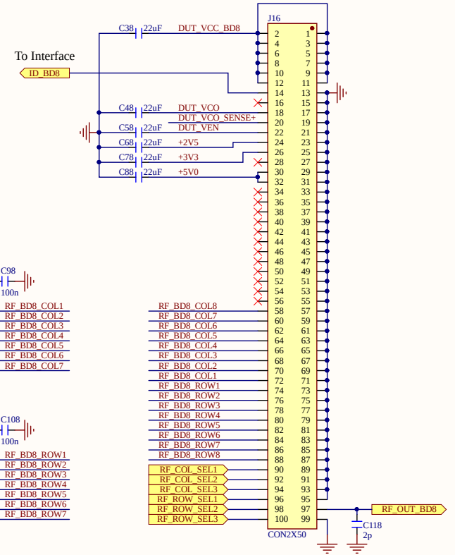
第八层8x8 DUT频率输出 To H-9220 Backplane Board - Interface
