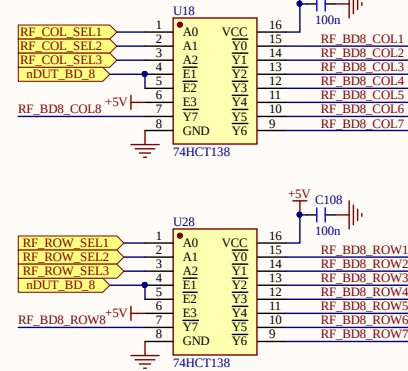
多路复用器 第八层8x8 DUT行列选通控制信号 From H-9220 Backplane Board - Interface
