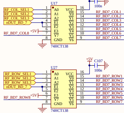
多路复用器 第七层8x8 DUT行列选通控制信号 From H-9220 Backplane Board - Interface
