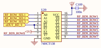
多路复用器 第九层8x8 DUT行列选通控制信号 From H-9220 Backplane Board - Interface
