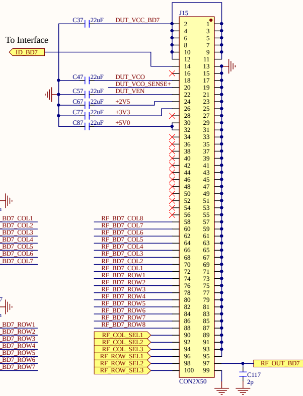
第七层8x8 DUT频率输出 To H-9220 Backplane Board - Interface
