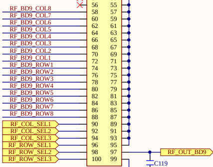
第九层8x8 DUT频率输出 To H-9220 Backplane Board - Interface
