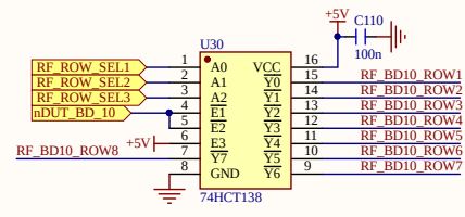
多路复用器 第十层8x8 DUT行列选通控制信号 From H-9220 Backplane Board - Interface
