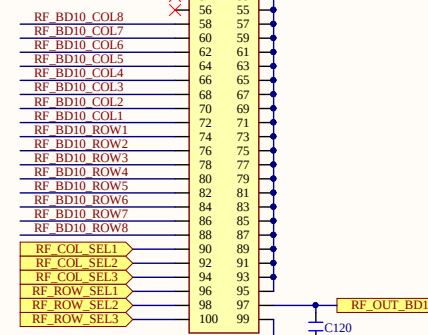
第十层8x8 DUT频率输出 To H-9220 Backplane Board - Interface
