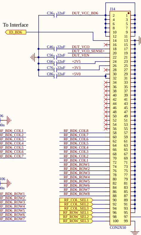
第六层8x8 DUT频率输出 To H-9220 Backplane Board - Interface
